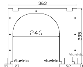
CAA36
