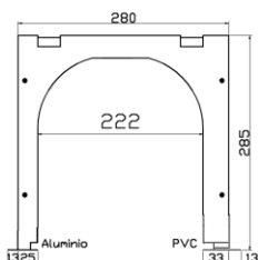
CAA28
