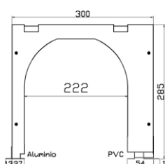
CAA30
