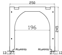
CAB25
