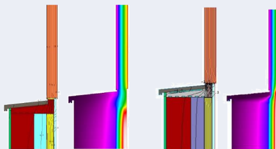
Sección lateral
