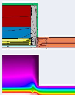
Sistema AISLABLOCK®, 67mm
